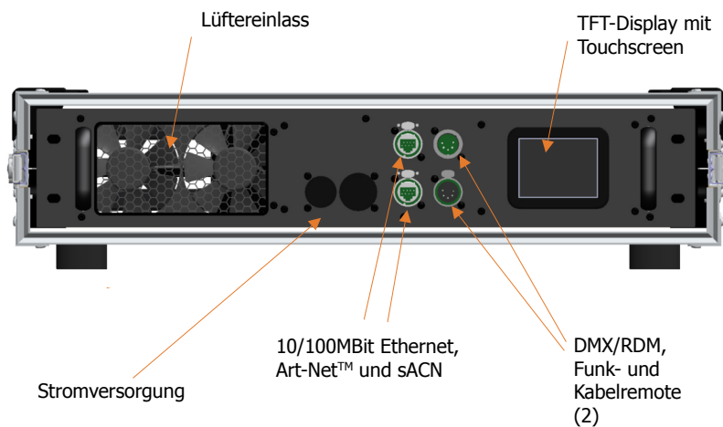
Rückansicht
